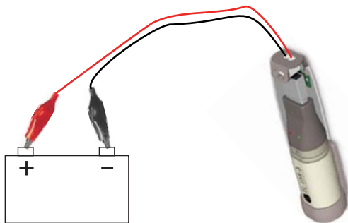
Enregistrement de la tension d'une pile
